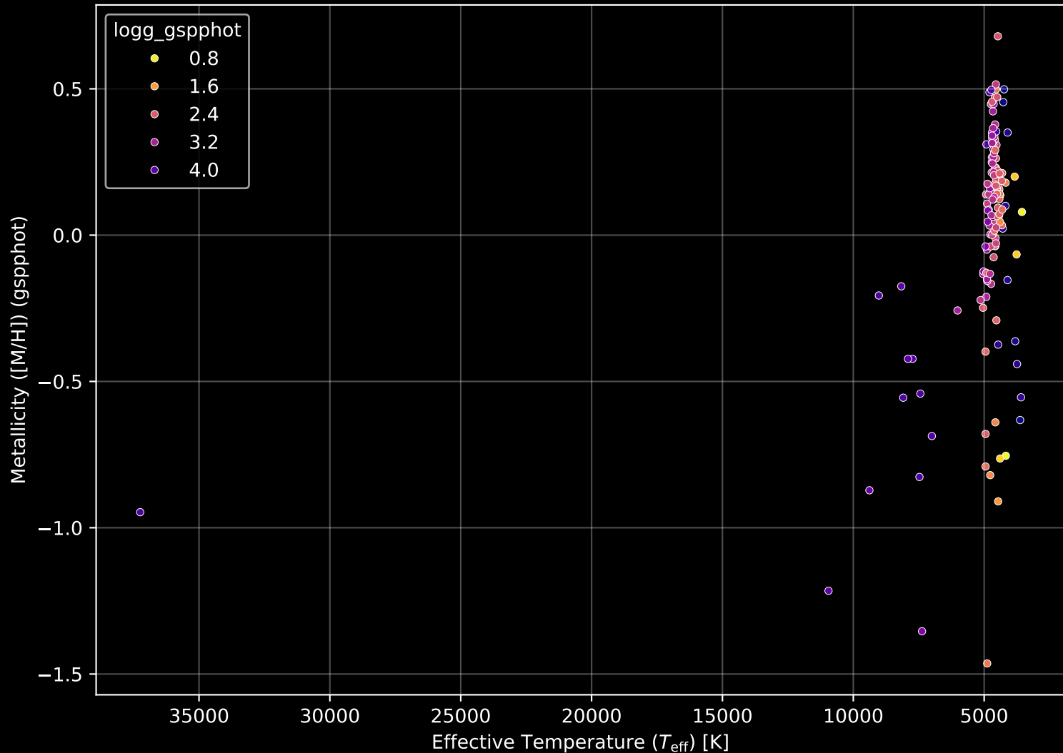
APOGEE DR17 Field: [SGRC-3] Stellar Population Parameters (n= 145)
